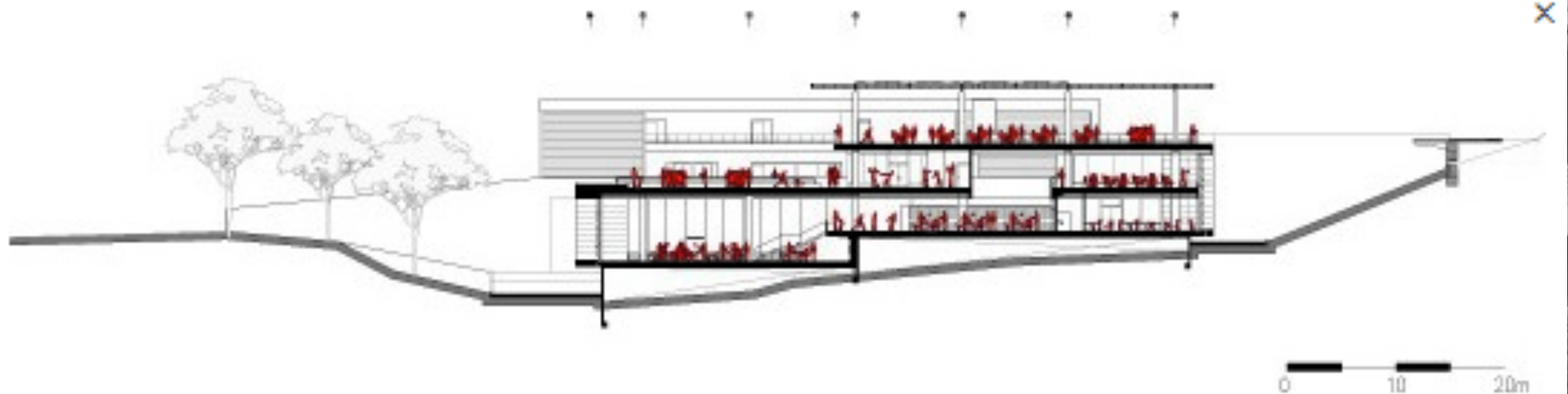
Biblioteca Tomás Carrasquilla / Sección a-a
